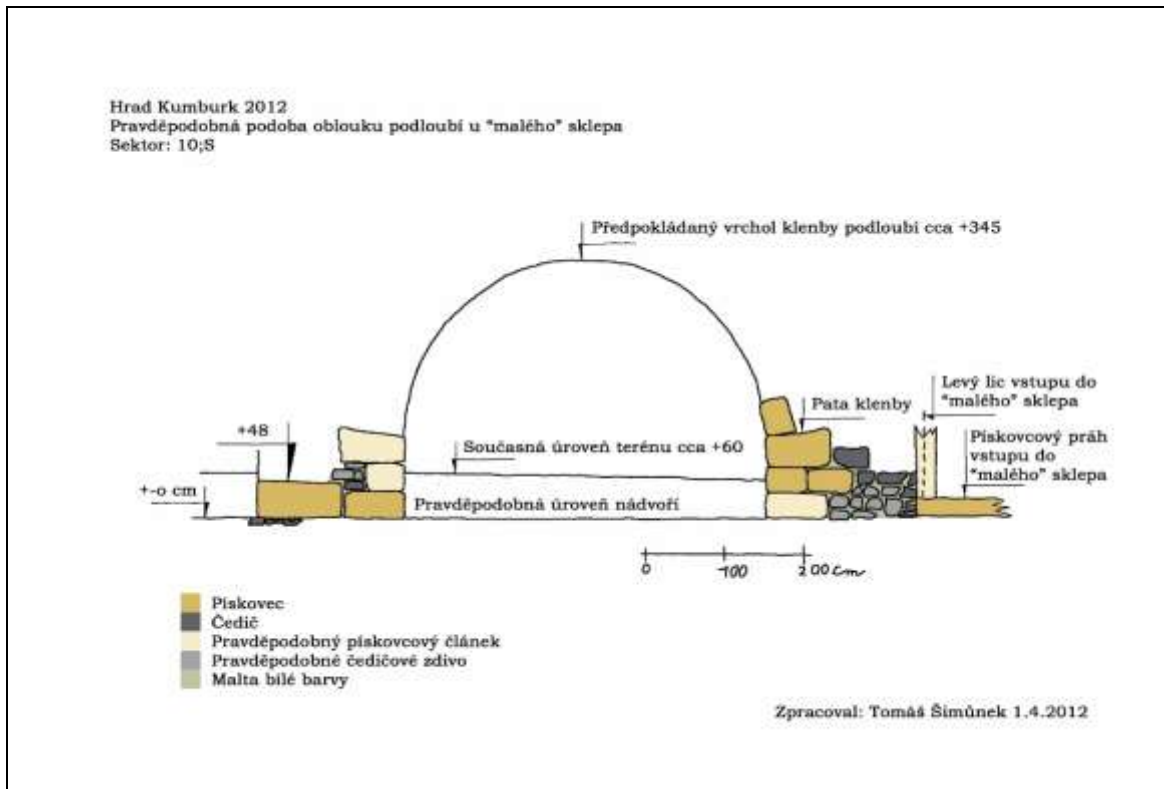
(Kumburk – pravděpodobná podoba oblouku podloubí u malého sklepa)
