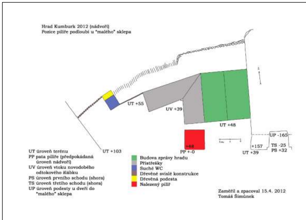
(Kumburk – torzo pilíře u malého sklepa - zaměření)
